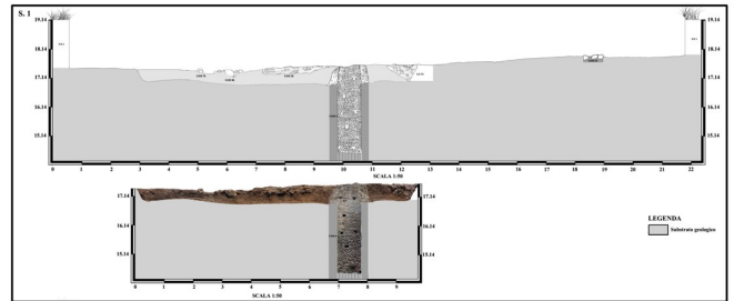
Fig. 3 - Pomezia (Rm) - Via Pratica di Mare 45. Sezione stratigrafica prospettica e ortofoto del pozzo
